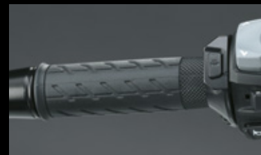
Griffheizung 57100-25810-000 Bietet drei verschiedene Heizstufen. Für höchsten Komfort wird die gesamte Oberfläche beheizt.
