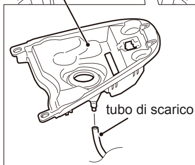
coperchio della scatola del casco
