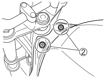
(SV650)
