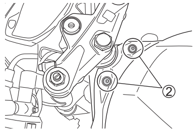
(SV650X)
