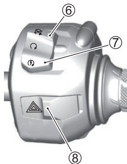
RECHTE LENKERARMATUR
