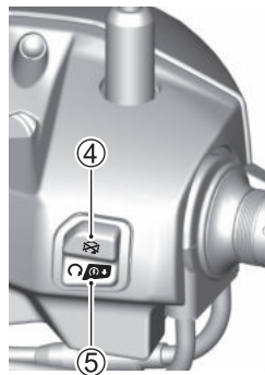
RECHTE LENKERARMATUR
