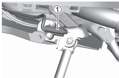
① Seitenständer-/Zündkreisverriegelungsschalter
